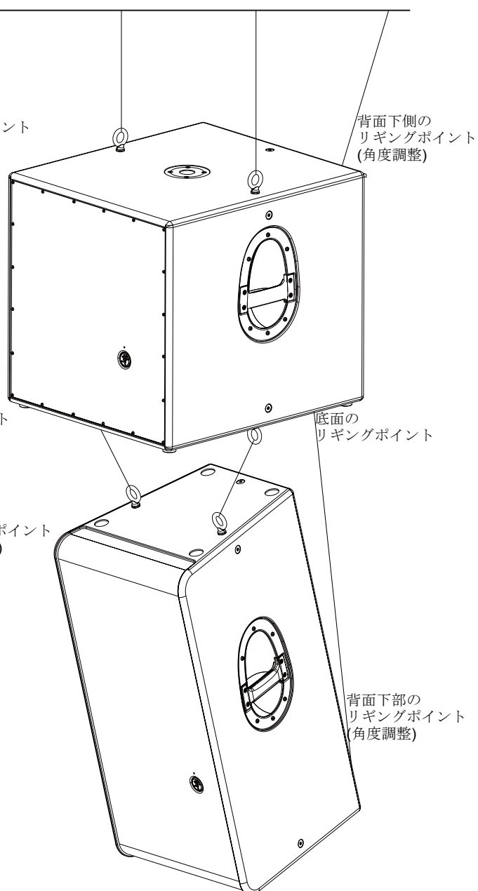
HD1801とHD531を垂直に吊った場合
