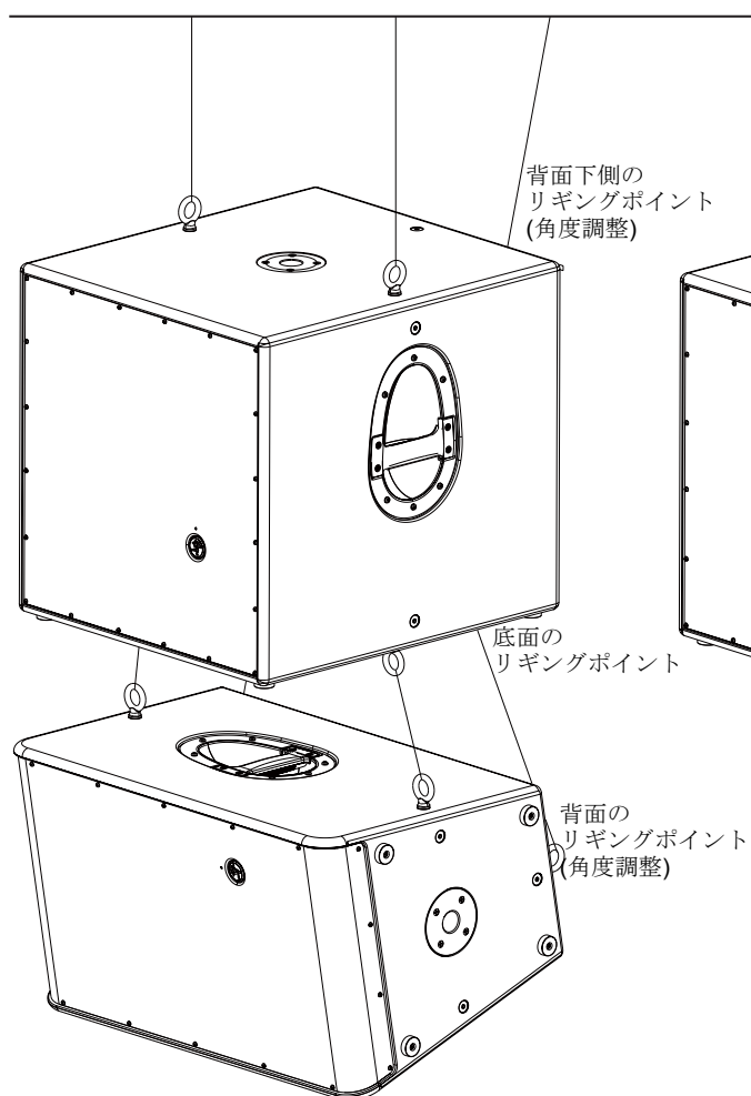
HD1801とHD521を垂直に吊った場合
