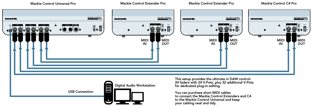
Hookup 1: USB
