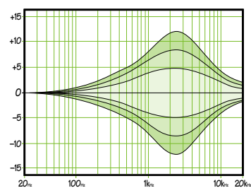
Mid EQ
