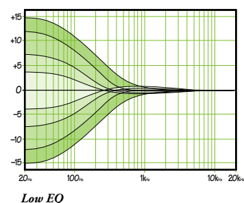
Low EQ
