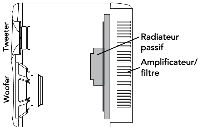
Figure 1. - Vue de coupe du HR824 MK2
