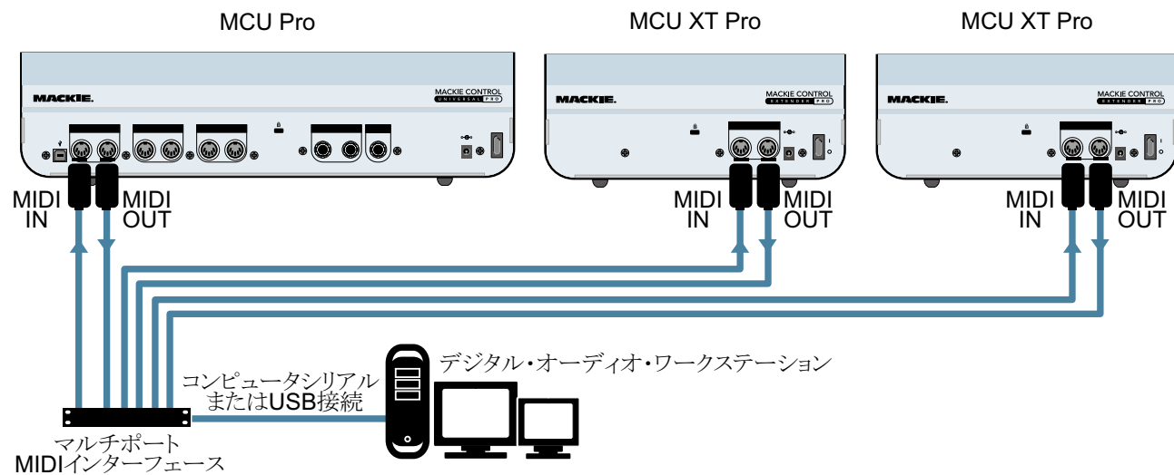
接続図 2 MIDI
