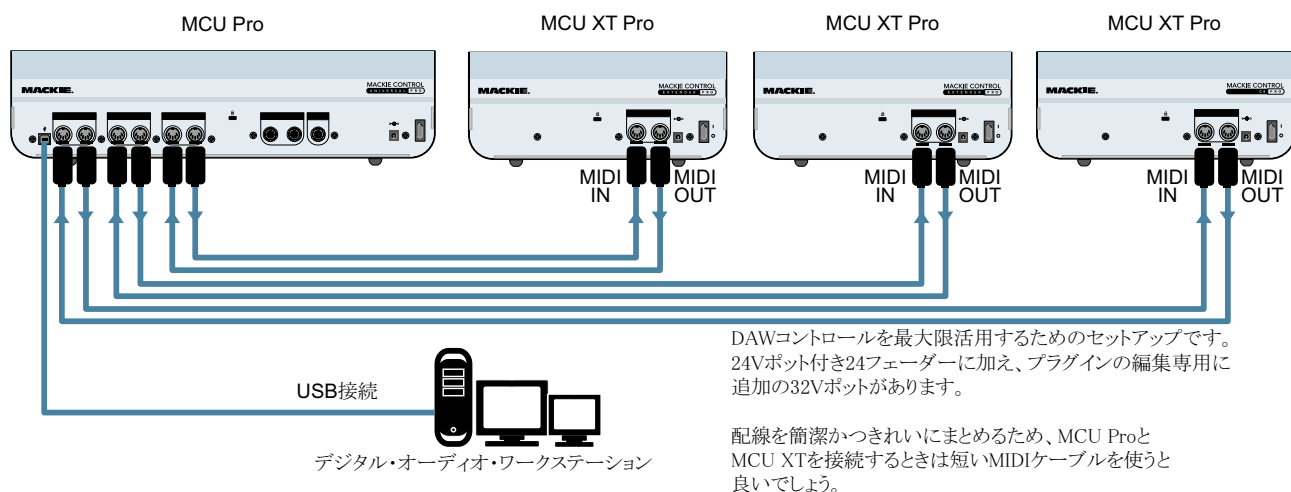
接続図 1 USB
