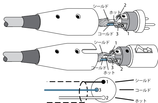
図 A: XLR コネクター
