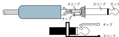
図 C: TS プラグ
