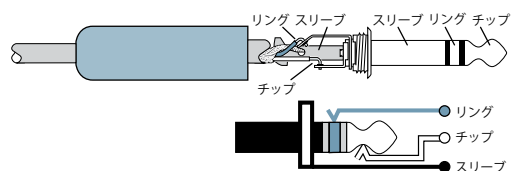
図 B: 1/4インチTRSプラグ
